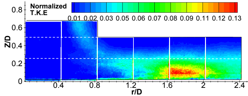
(d). Distribution of turbulence kinetic energy (T.K.E)
